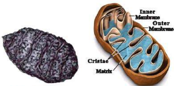
Mitochondria
