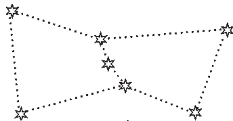
चित्र 1.4 मृग या ओरायन तारामण्डल
