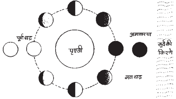
चित्र 1.10 चन्द्रमा की कलाएँ, पृथ्वी और सूर्य के सापेक्ष इसकी स्थिति में परिवर्तन के कारण होती हैं।
