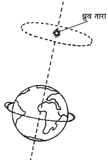
चित्र 1.2 ध्रुव तारा पृथ्वी के घूर्णन अक्ष के समीप स्थित है।
