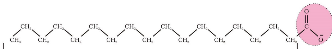
सोडियम स्टीरेट ( C_{17}H_{35}COO^- Na^+ )
