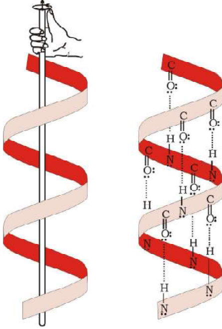
चित्र 14.1— प्रोटीन की \alpha -कुण्डलित संरचना
