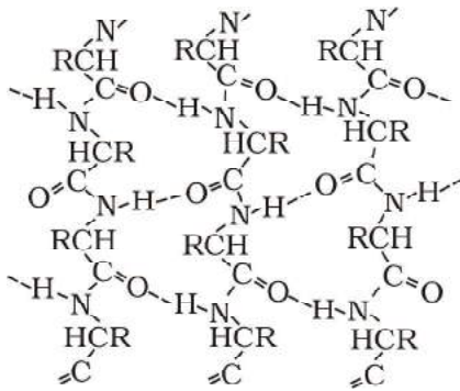
चित्र 14.2— प्रोटीन की \beta -शीट संरचना
