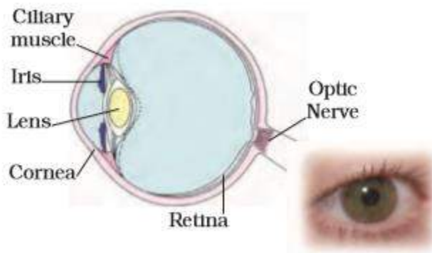
Fig. 16.14 : Human eye
