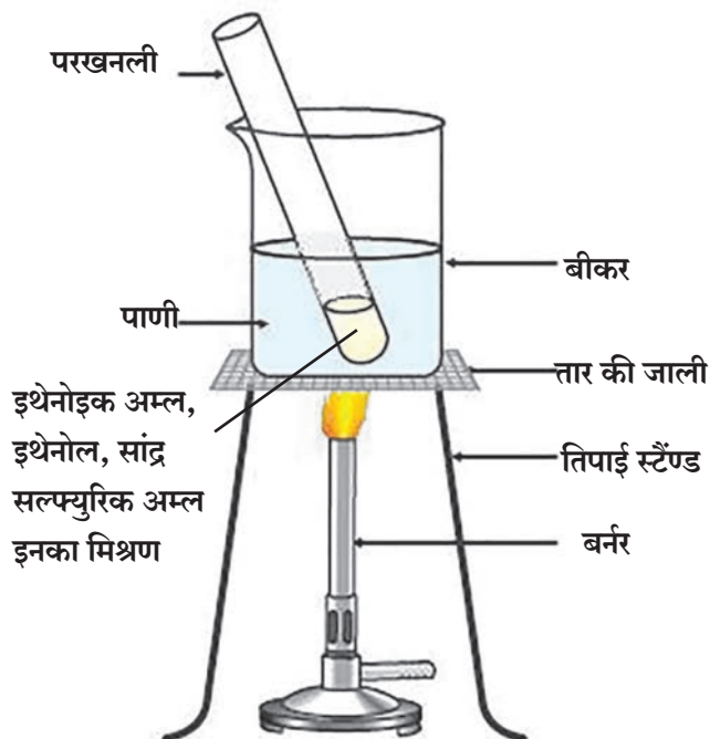
9.25 ईस्टरीकरण अभिक्रिया
