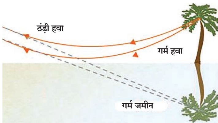
6.5 मृग मरीचिका
