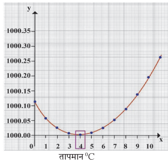
5.4 पानी के तापमान तथा आयतन का आलेख
