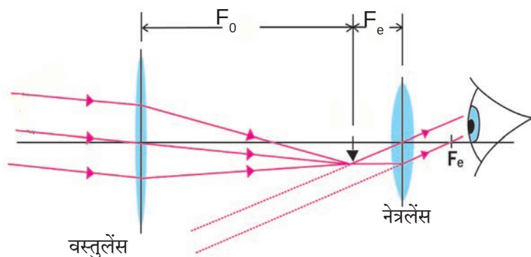
7.18 अपवर्तनी दूरदर्शी
