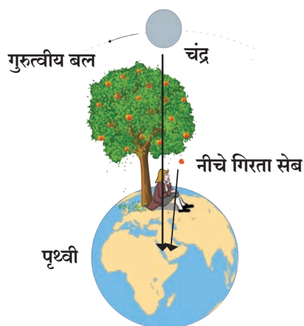
1.1 गुरुत्वाकर्षण बल की कल्पना और सेब एवं चंद्रमा पर लगनेवाला गुरुत्वीय बल
