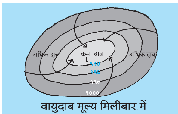
आकृति ५.७ : चक्रवात
