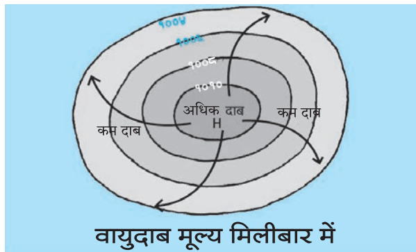
आकृति ५.९ : प्रतिचक्रवात
