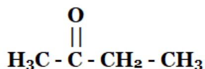
Butanone
