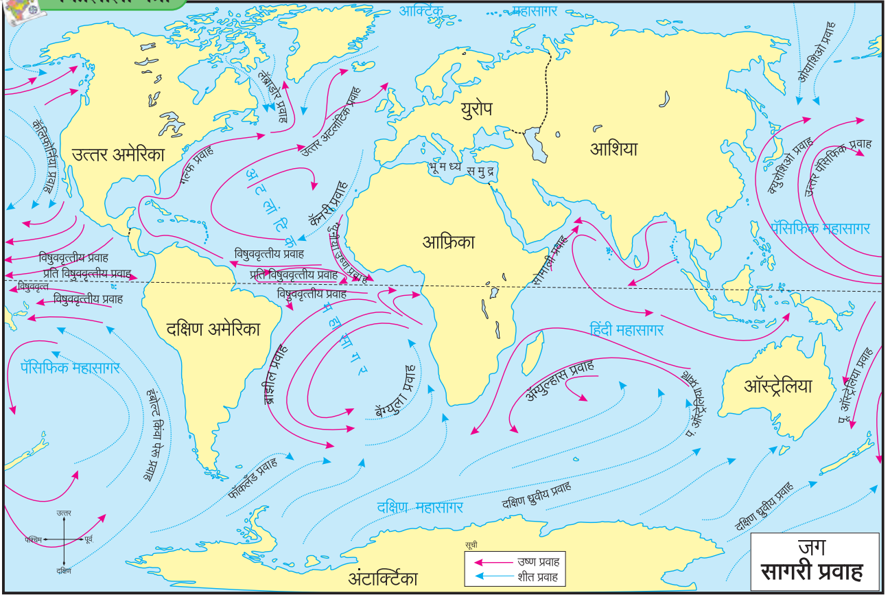
आकृती ५.४ : सागरी प्रवाह
