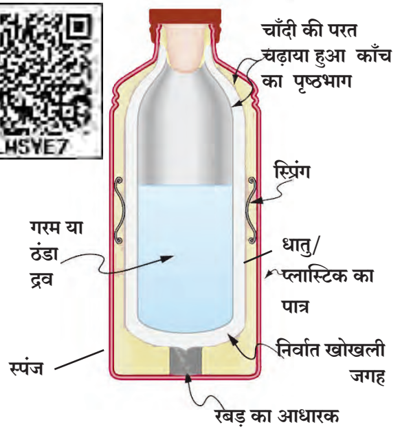
9.8 थर्मस फ्लास्क
