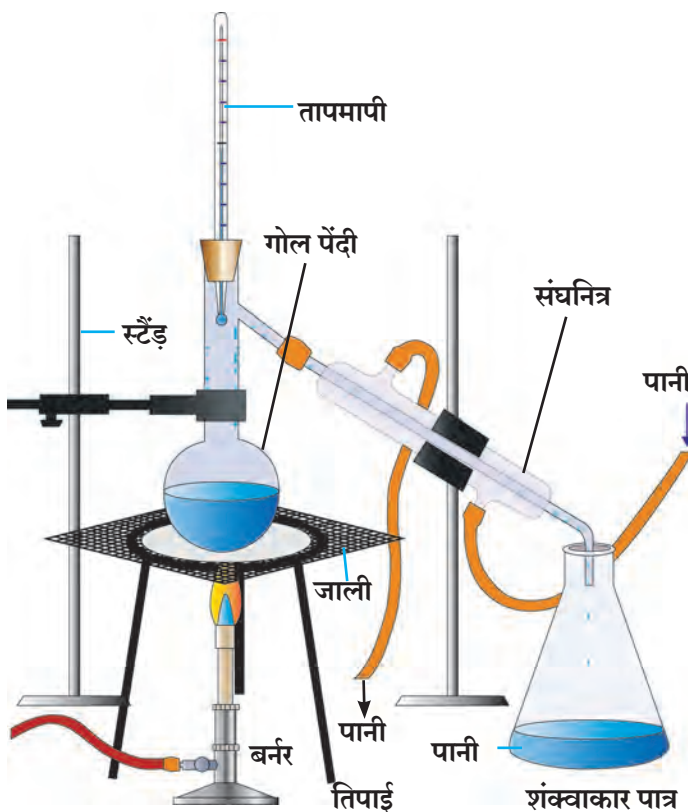
14.4 आसवन विधि
