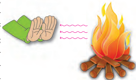
9.5 विकिरण
