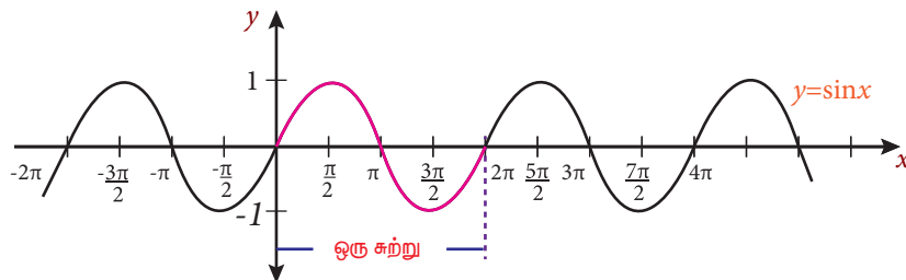
படம் 3.13 : y = \sin x
