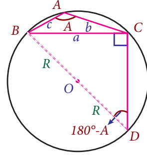
\angle A ஒரு விரிகோணம்
