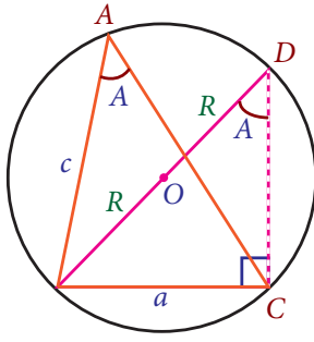
\angle A ஒரு குறுங்கோணம்
