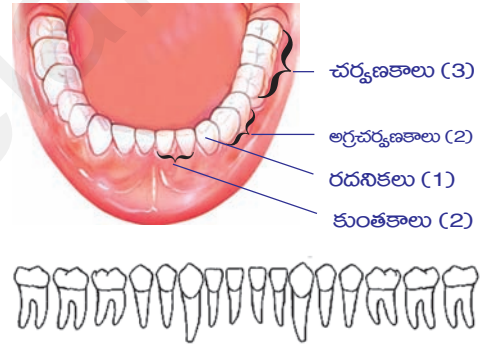
పటం-3: దంతాల అమరిక
