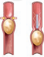
పటం-5: సైకిల్ ట్యూబ్ లో బంగాళదుంప
