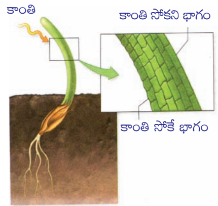
పటం-20: కణాల వంగడం
