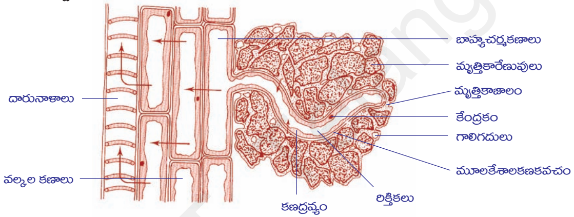
పటం-16: మృత్తికాజాలం మూలకేశాలతో సంబంధాన్ని చూపే వేరు నిలుపుకోత
