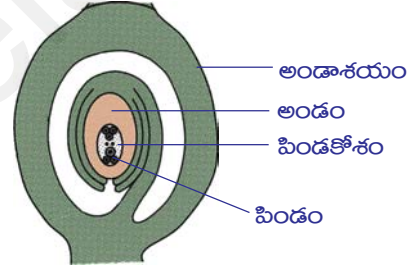
పటం-20: అండం - నిర్మాణం
