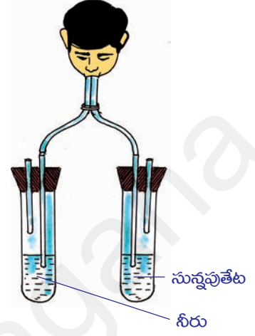
పటం-3: కార్బన్ డై ఆక్సైడ్ ఉనికిని గుర్తించుట
