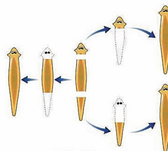
పటం-5: ఫ్లనేరియాలో పునరుత్పత్తి
