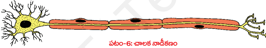
పటం-6: చాలక నాడీకణం
