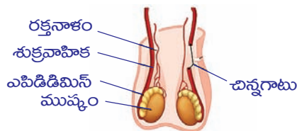
వాసెక్టమి-శుక్రవాహికను కత్తిరించి ముడివేయడం
