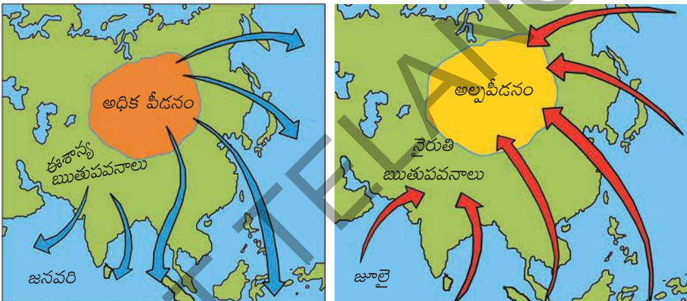
తిరోగమన ఋతుపవనాలు చిత్రం 4.3 : పీడనం, ఋతుపవనాలు
